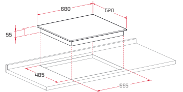
W 858 CAT EI Ankastre Cam Ocak 70 cm / 5 Gözü Gazlı (4 Gaz+1 Wok)
