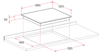
858 CAT EI Ankastre Cam Ocak 70 cm / 5 Gözü Gazlı (4 Gaz+1 Wok)
