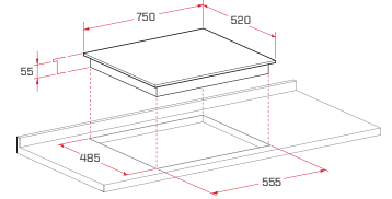
WL 858 CAT DI Ankastre Cam Ocak 75 cm / 5 Gözü Gazlı (4 Gaz+1 Wok)
